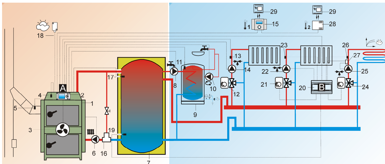
Obr. 9 Schéma s akumulční nádrží – s modulem B² , kde: 1 - kotel, 2 – regulátor, 3 – ventilátor, 4 – čidlo teploty kotle, 5 – čidlo teploty spalin, 6 – čerpadlo kotle, 7 – akumulace, 8 – čerpadlo TUV, 9 – zásobník TUV, 10 – čerpadlo cirkulace TUV, 11 – čidlo TUV, 12 – pohon směšovače, 13 – čidlo směšovače, 14 – čerpadlo směšovače, 15 – pokojový panel SPARKSTER s funkcí termostatu, 16 – termostatický, směšovací ventil pro ochrnu zpátečky, nebo Laddomat, 17 – horní čidlo akumulace, 18 – venkovní čidlo teploty, 19 – dolní čidlo akumulace, 20 – modul B, 21 – pohon směšovače, 22 – čerpadlo směšovače, 23 – čidlo směšovače, 24 – pohon směšovače, 25 – čerpadlo směšovače, 26 – čidlo směšovače, 27 – mechanický bezpečnostní termostat, pro vypnutí čerpadla podlah.vytápění, 28 – pokojové čidlo panelu SPARKSTER, 29 – běžný pokojový termostat (místo panelu SPARKSTER).
