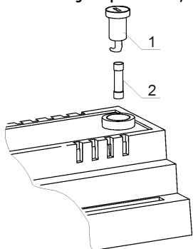
Obr. 26 Výměna pojistky, kde: 1 – pojistka, 2 – držák pojistky
