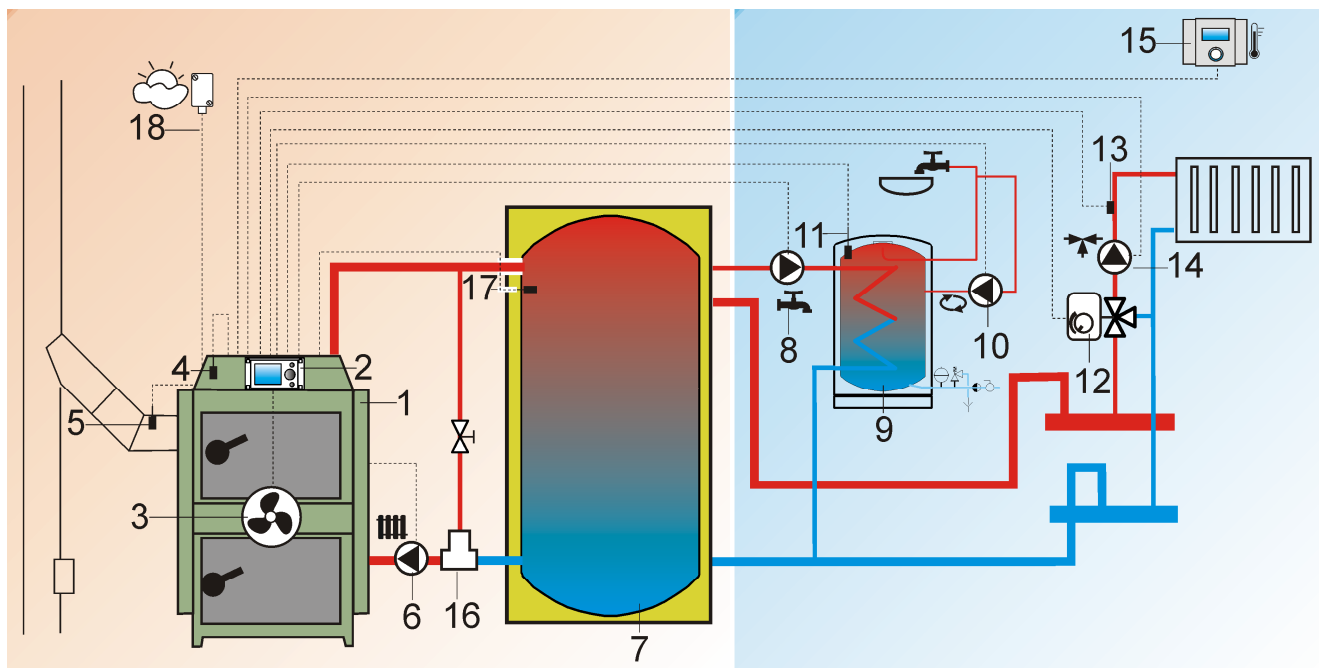
Obr. 8 Schéma s akumulční nádrží – bez dodatkových modulů , kde: 1 - kotel, 2 - regulátor, 3 - ventilátor, 4 - čidlo teploty kotle, 5 - čidlo teploty spaliny, 6 - čerpadlo kotle, 7 - akumulace, 8 - čerpadlo TUV, 9 - zásobník TUV, 10 - čerpadlo cirkulace TUV, 11 - čidlo TUV, 12 - pohon směšovače, 13 - čidlo směšovače, 14 - čerpadlo směšovače, 15 - pokojový panel SPARKSTER s funkcí termostatu, 16 - termostatický, směšovací ventil pro ochrnu zpátečky, nebo Laddomat, 17 - horní čidlo akumulace, 18 - venkovní čidlo teploty
