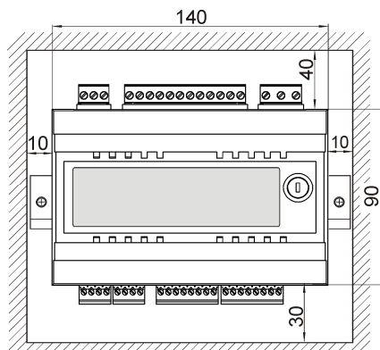
Obr. 15 Podmínky pro instalaci modulu
